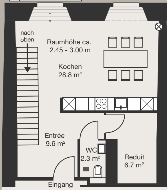
Grundriss 4. Obergeschoss
