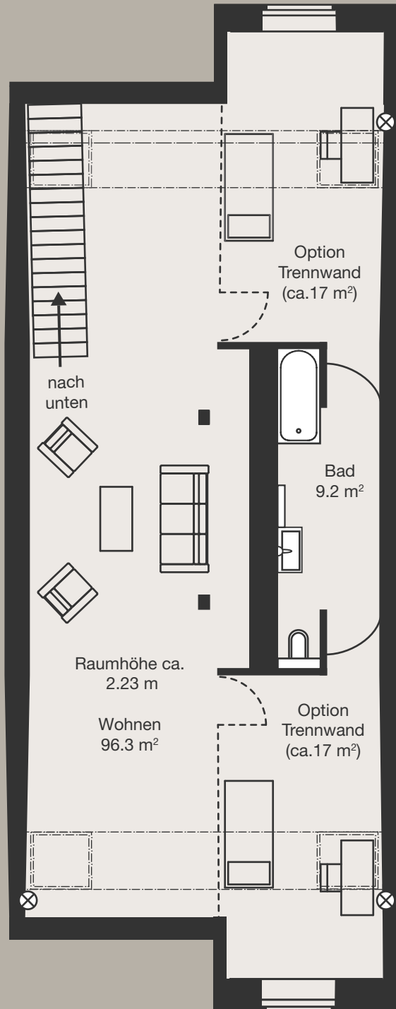
Grundriss 1. Dachgeschoss
