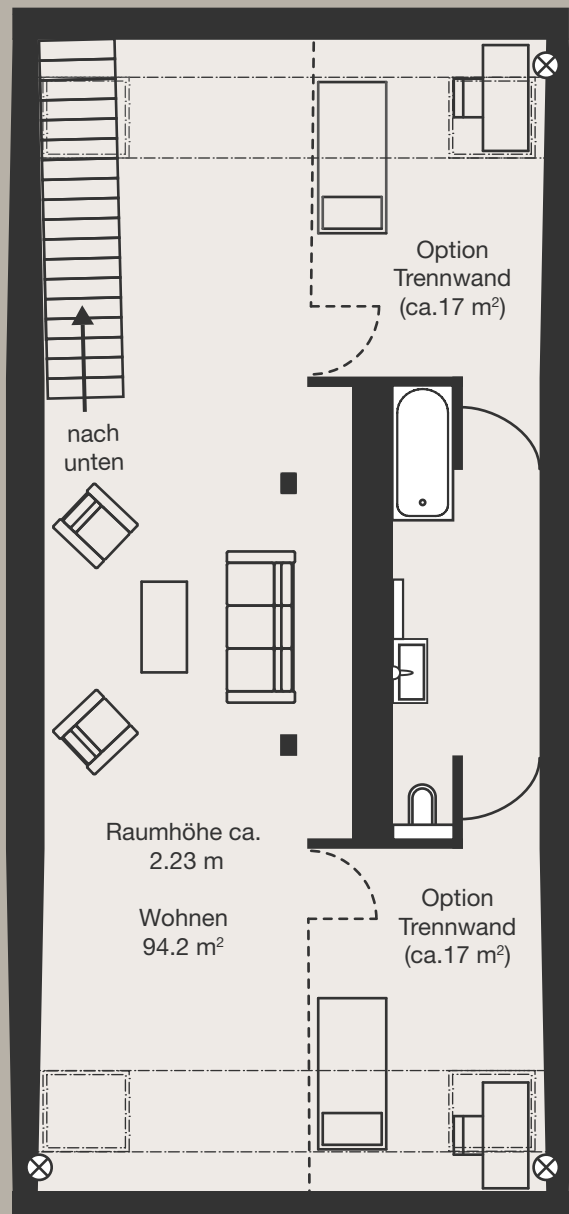
Grundriss 1. Dachgeschoss
