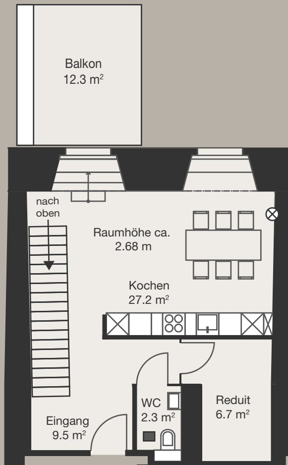
Grundriss 1. Obergeschoss
