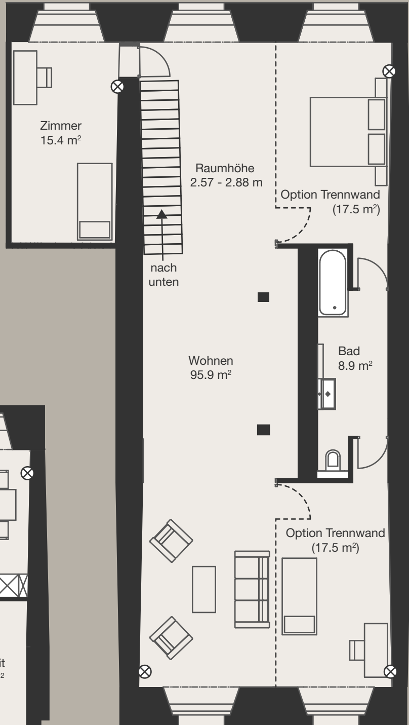
Grundriss 2. Obergeschoss
