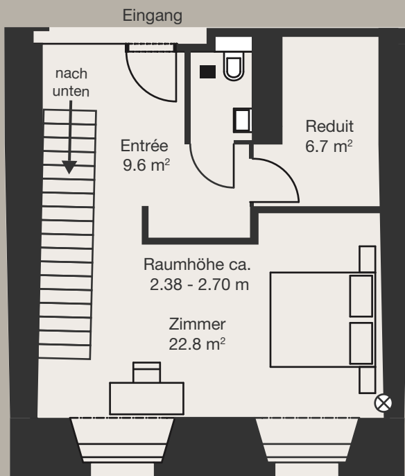
Grundriss 1. Obergeschoss
